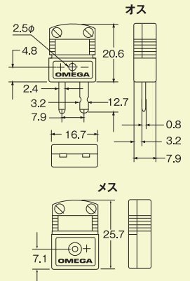
〈SMPW 寸法図〉:単位mm
